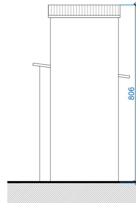
PROSPETTO OVEST
