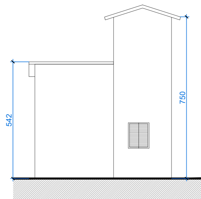
PROSPETTO NORD
