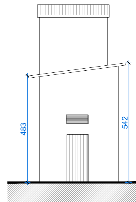
PROSPETTO EST
