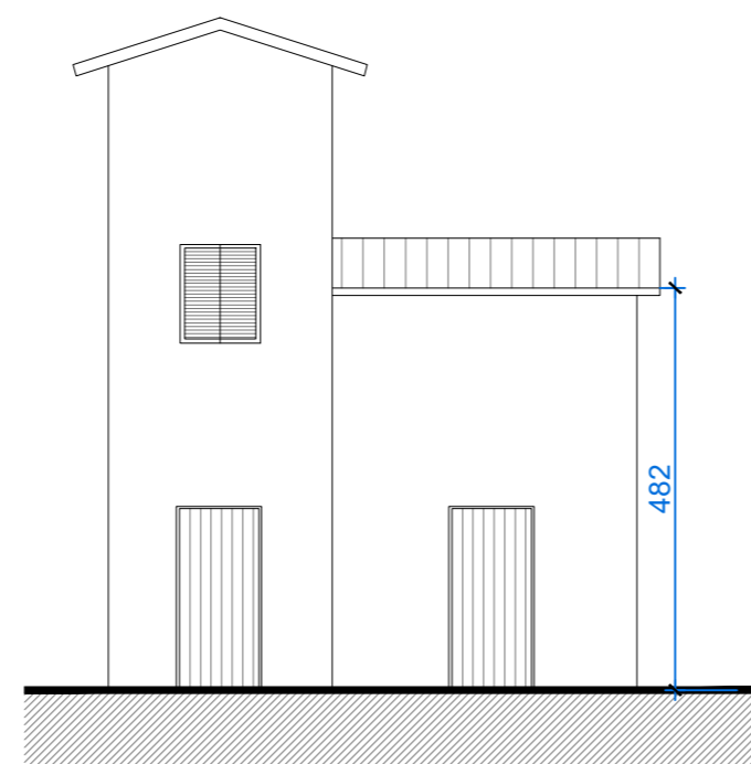
PROSPETTO SUD
