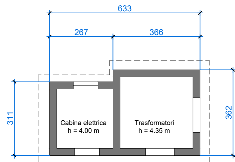
PIANTA PT
