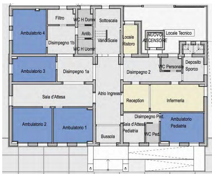
1. Pianta del piano Terra
